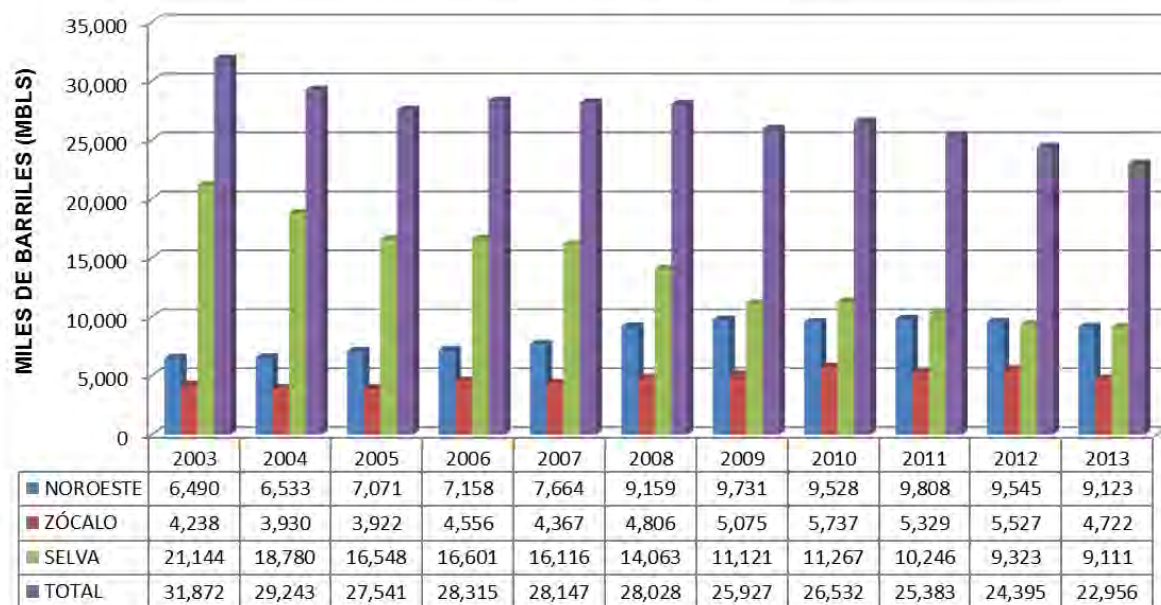
PRODUCCIÓN FISCALIZADA DE PETROLEO 2003 - 2013
