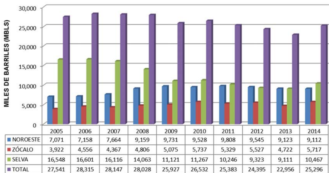
Gráfico N° 31 PRODUCCIÓN FISCALIZADA DE PETROLEO: 2005 - 2014
