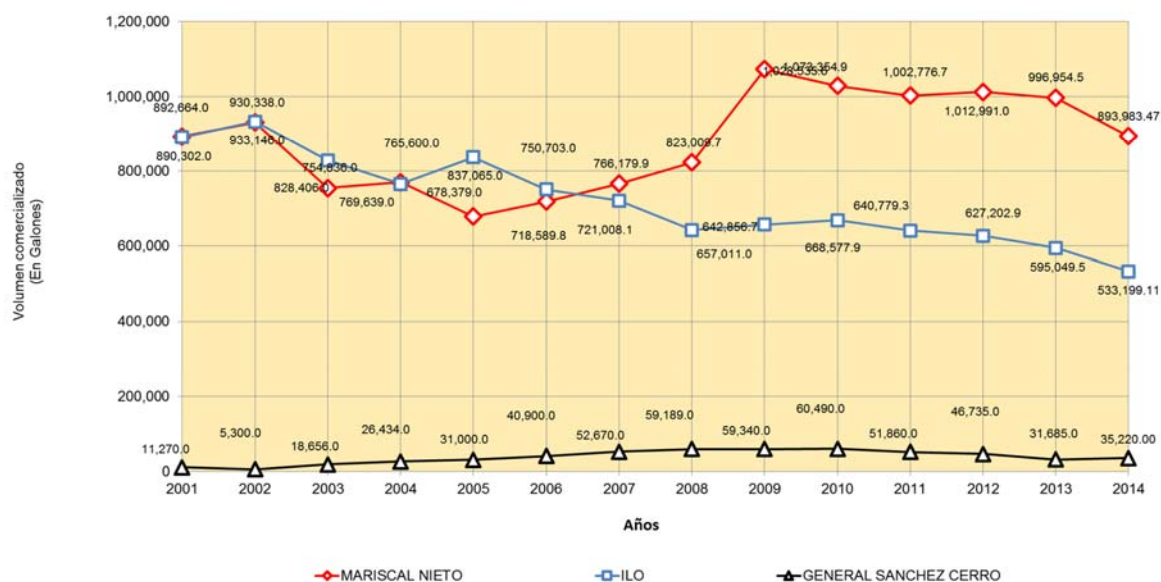
Gráfico N° 07: REGION MOQUEGUA: VOLUMEN COMERCIALIZADO DE GASOLINA 84 OCT. POR PROVINCIAS: 2001- 2014
