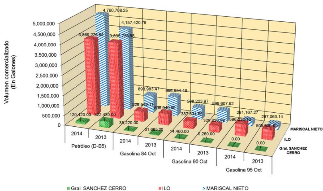
Grafico N° 20 REGION MOQUEGUA: VARIACIÓN DEL VOLUMEN COMERCIALIZADO SEGUN TIPO DE COMBUSTIBLES LIQUIDOS Y POR PROVINCIAS: 2014 / 2013
