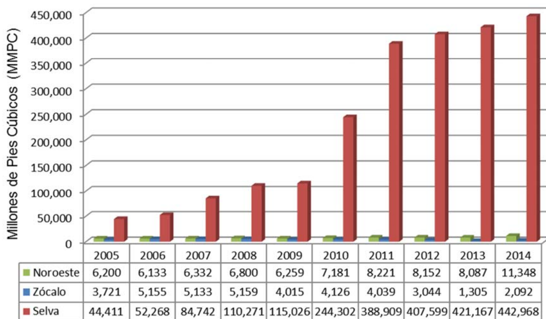
Gráfico N° 33 PRODUCCIÓN FISCALIZADA DE GAS NATURAL: 2005 - 2014
