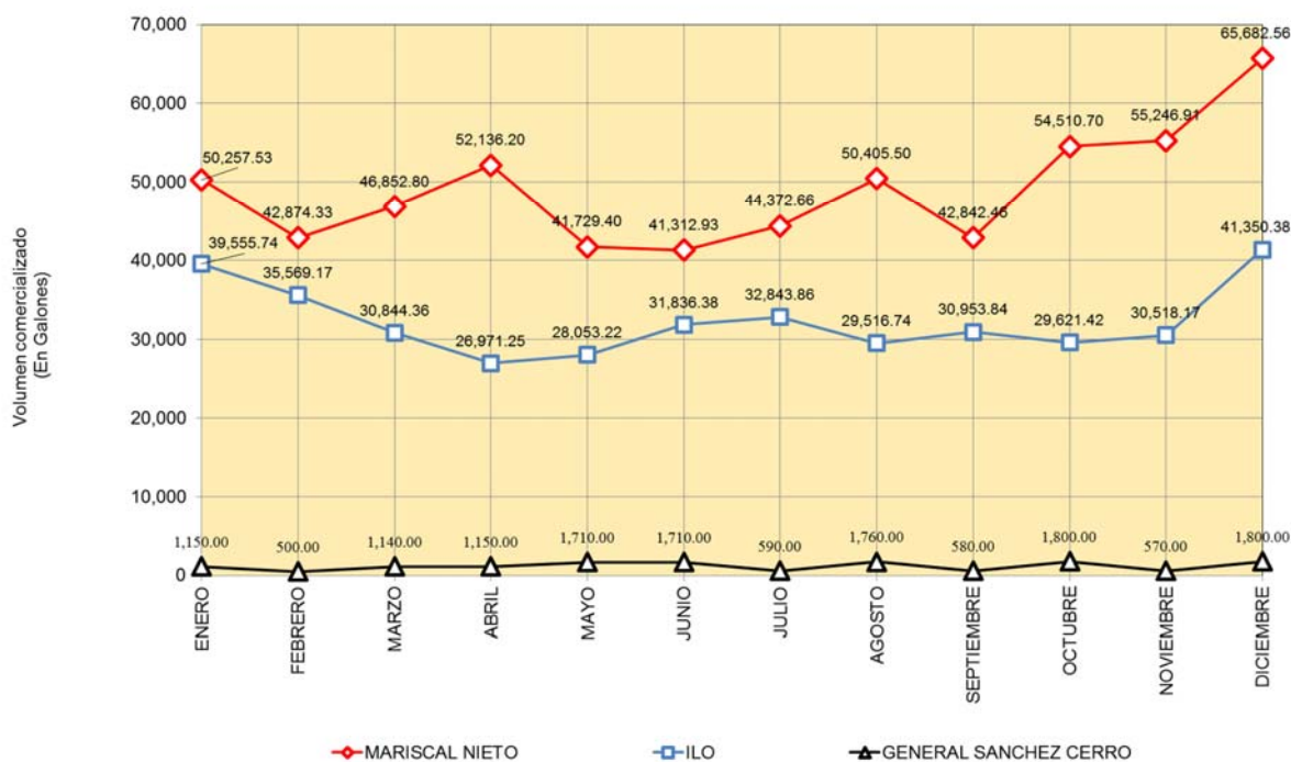
Grafico N° 09 REGION MOQUEGUA: VOLUMEN COMERCIALIZADO POR PROVINCIA DE GASOLINA 90 OCTANOS - 2014
