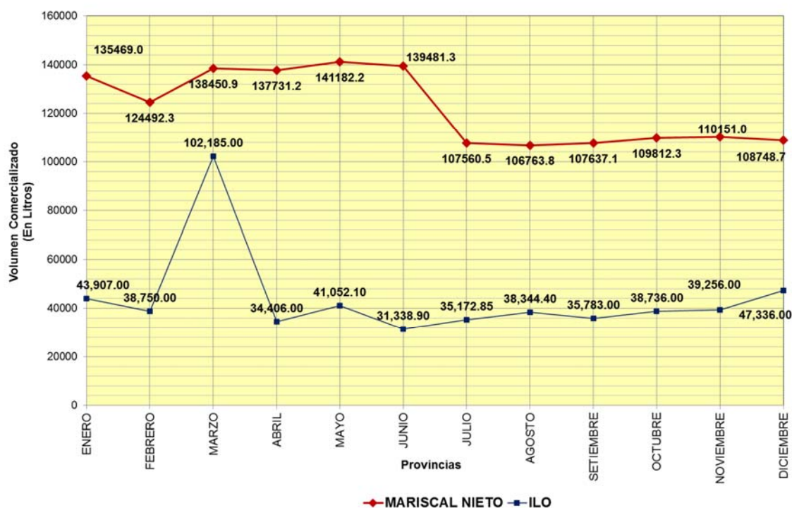
Grafico N° 21 REGION MOQUEGUA: VOLUMEN COMERCIALIZADO DE GAS LICUADO DE PETROLEO POR PROVINCIAS: 2014
