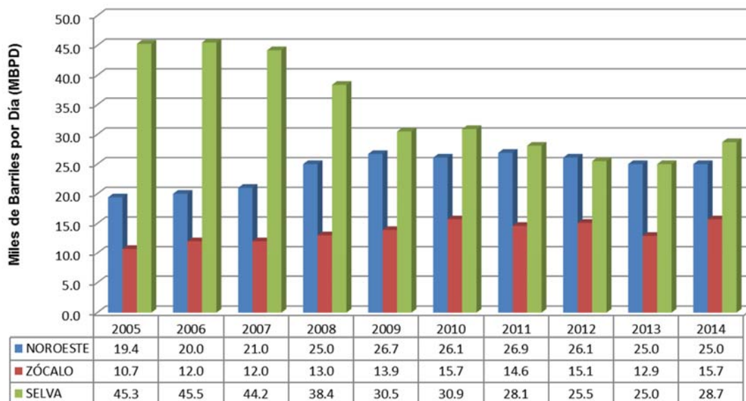
Gráfico N° 32 PRODUCCIÓN FISCALIZADA DE PETROLEO: 2005 - 2014
