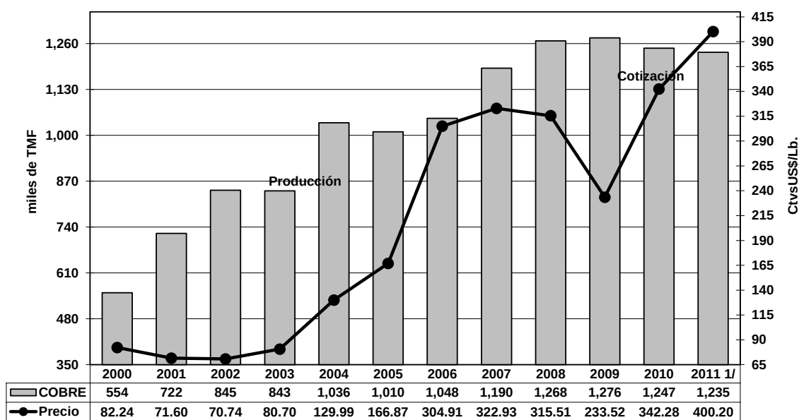
GRÁFICO N° 17 PERÚ: PRODUCCIÓN DE COBRE Y COTIZACIÓN 2000 - 2011
