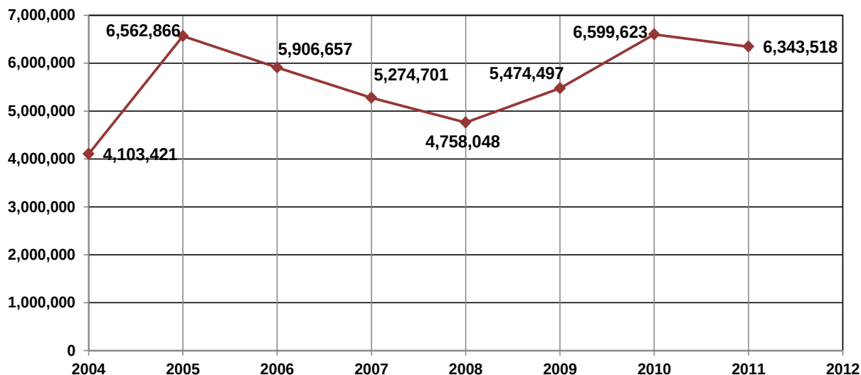
Gráfico N° 7 MOQUEGUA: PRODUCCIÓN TOTAL DE ORO, 2004- 2011 (Toneladas métricas)
