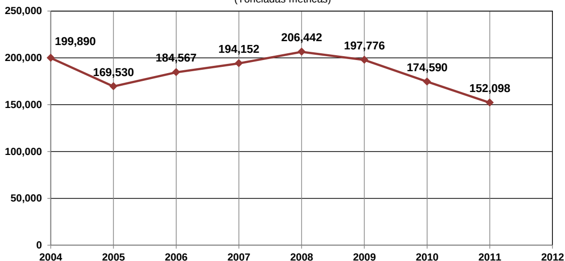
Gráfico N° 6 MOQUEGUA: PRODUCCIÓN TOTAL DE COBRE, 2004- 2011 (Toneladas métricas)
