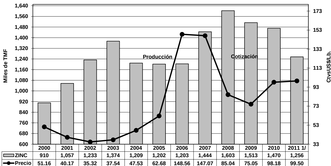
GRÁFICO N° 19 PERÚ: PRODUCCIÓN DE ZINC Y COTIZACIÓN 2000 - 2011
