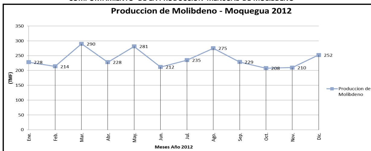
Gráfico N°4 COMPORTAMIENTO DE LA PRODUCCIÓN MENSUAL DE MOLIBDENO
