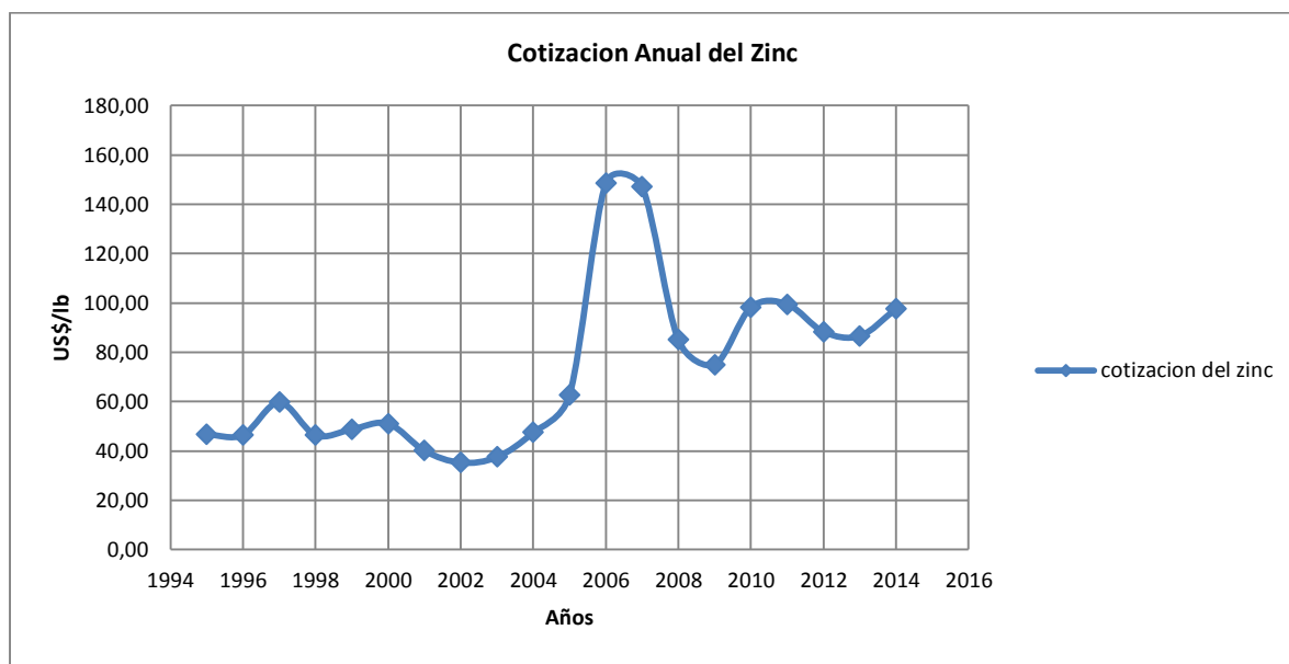
Grafico N°17 MOQUEGUA: COTIZACIÓN ANUAL PROMEDIO DE ZINC (US$/lb.)
