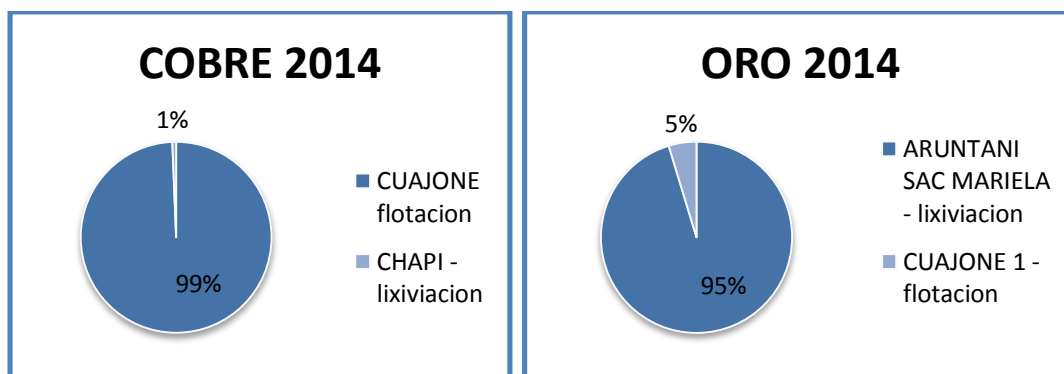
Grafico N°7 MOQUEGUA: PORCENTAJE DE PRODUCCIÓN POR UNIDAD DE COBRE Y ORO, 2014
