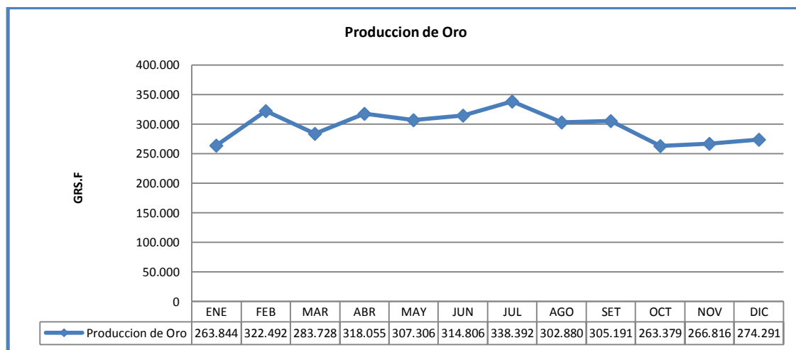
Grafico N°2 COMPORTAMIENTO DE LA PRODUCCIÓN MENSUAL DE ORO 2014
