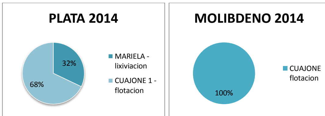
Grafico N°10 MOQUEGUA: PORCENTAJE DE PRODUCCIÓN POR UNIDAD DE PLATA Y MOLIBDENO, 2014
