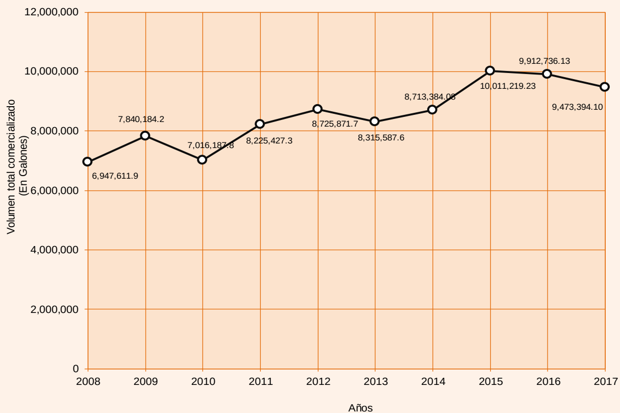
Gráfico N° 04 REGION MOQUEGUA: VOLUMEN TOTAL COMERCIALIZADO DE DIESEL B5: 2008 - 2017
