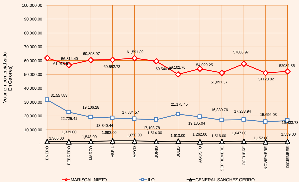
Gráfico N° 05 REGION MOQUEGUA: VOLUMEN COMERCIALIZADO DE GASOLINA 84 OCT. POR PROVINCIAS: 2017
